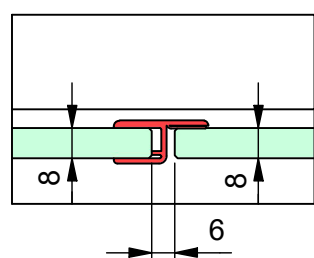
b) mit Dichtprofil 8856KU0-8
