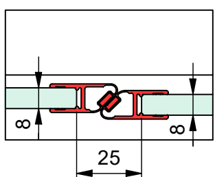
a) mit Dichtprofil 8852KU0-8
