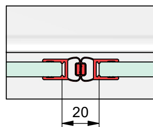
c) mit Dichtprofil 8850KU0-8
