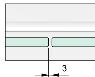
d) ohne Dichtprofil
