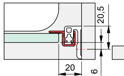
c) mit Dichtprofil 8855KU0-8 und Türanschlag-Trägerprofil 8880
