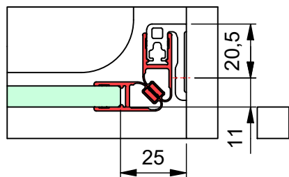
b) mit Dichtprofil 8851KU0-8 und Türanschlag-Trägerprofil 8880
