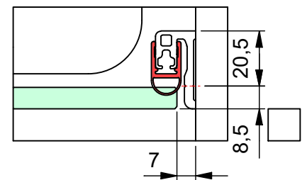
d) mit Dichtprofil 8861KU0-8 und Türanschlag-Trägerprofil 8880
