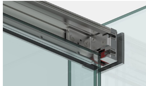
Ansicht am Seitenteil, Tür geöffnet view of side panel, door open
