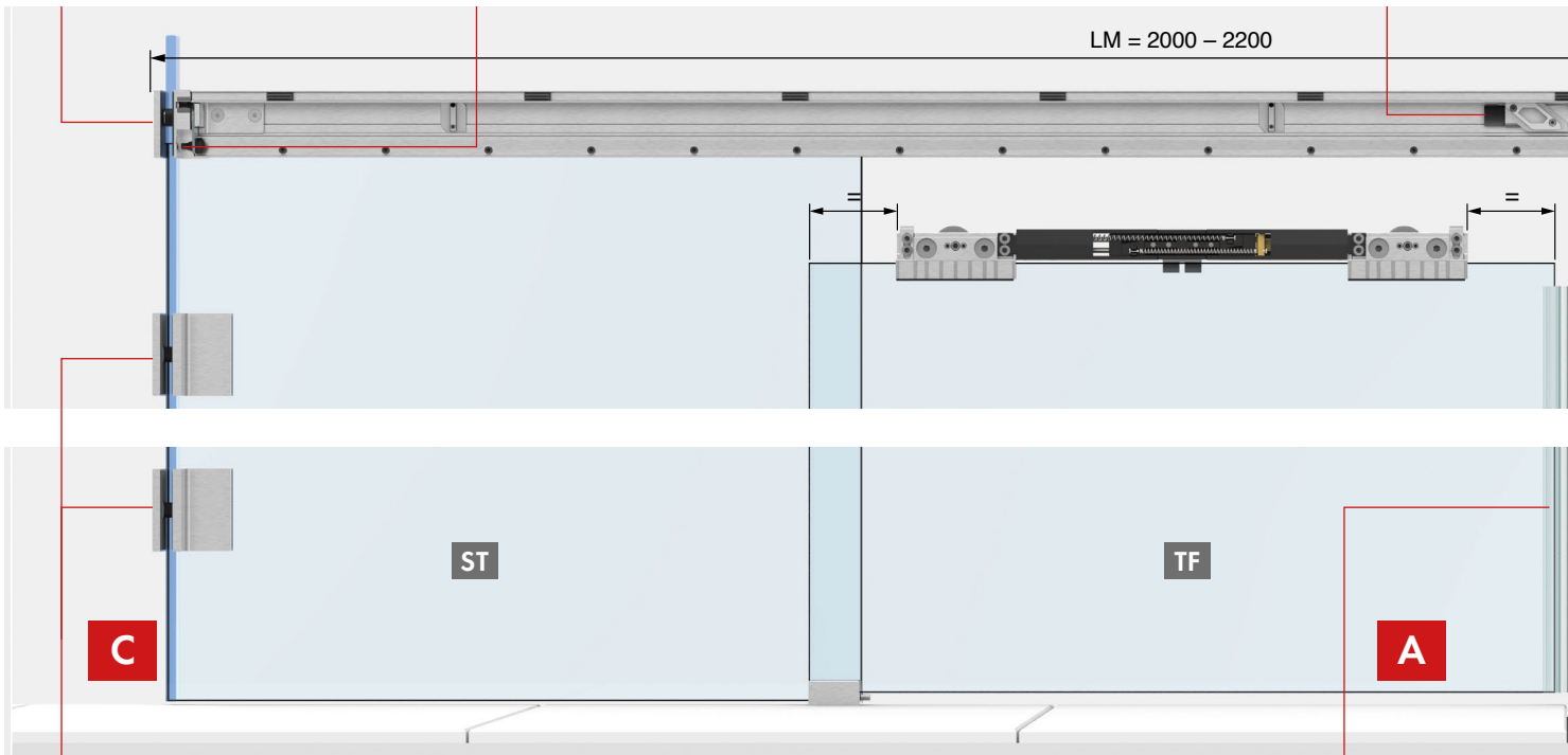
Glashalterung am Seitenteil glass bracket on the side panel Art.-Nr.: | art no.: 8822ZN_GRS/GLS
