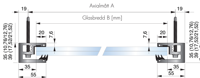
Möjlig glasdimensioner Typ P-01 / 7280
