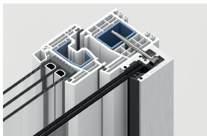
Fönsterkarmar av stålförstärkt PVC
