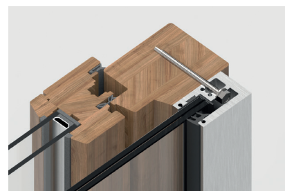
Träfönster och jämförbara träkonstruktioner
