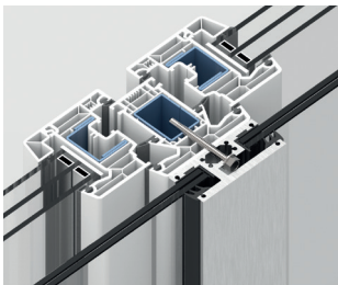
Art-Nr. 7282 Montageart K För PVC-fönster och kompositfönster PVC / aluminium med stålförstärkning (dold karminfästning)
