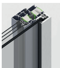
Art-Nr. 7280 Montagetyp A För aluminiumfönster (dold karminfästning)
