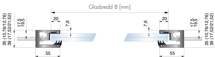
Möjliga glasdimensioner Typ P-02 / 7281
