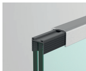
Kantskydd, U-profil av rostfritt stål A4 Art-Nr. 5022 Sid 12
