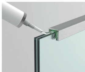
Kantskydd U-Profil av aluminium Art-Nr. 5023/5024/5026/5027 Sid 12
