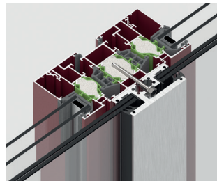
Art-Nr. 7282 Montageart A För aluminiumfönster (dold karminfästning), träfönster och kompositfönster trä / aluminium
