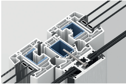
Fönsterkarm av stålförstärkt PVC
