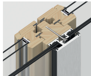
Art-Nr. 7282 Montageart A För aluminiumfönster (dold karminfästning), träfönster och kompositfönster trä / aluminium
