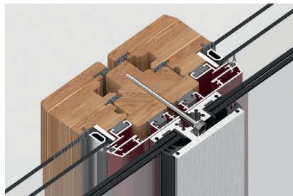
Kompositfönster trä / aluminium
