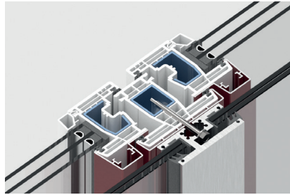
Kompositfönster PVC / aluminium med stålförstärkning
