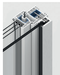
Art-Nr. 7280 Montagetyp K För PVC-fönster och kompositfönster PVC / aluminium med ställförstärkning (dold karminfästning)
