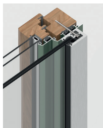
Art-Nr. 7280 Montagetyp A För träfönster och kompositfönster trä/aluminium (dold karminfästning)
