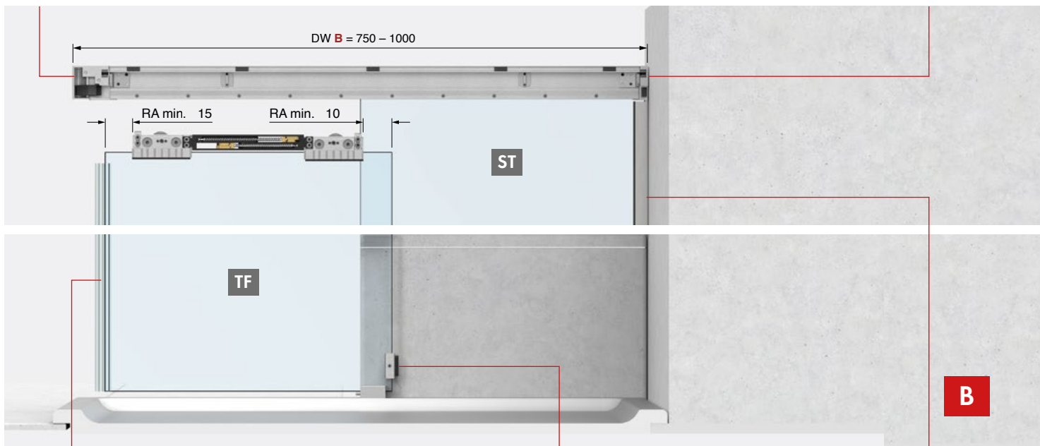
Support mural coté fixe Réf. Art.: 8822ZN_EL/ER
