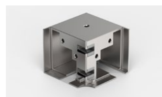
Raccord d'angle Panneau coulissant/Fixe Réf. Art.: 8822ZN_-EST90L
