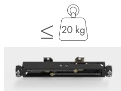
1 x Softstop 2 cotés (20 kg) Réf. Art.: 8822RAL7016-SSDD-20
