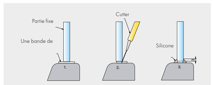
PVC souple pour parties fixes (100x80 mm, épaisseur 2 et 3 mm) Réf. Art.: 8870KU0
