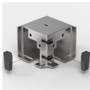
Raccord d'angle pour entrée d'angle (ouvrant/ouvrant) Réf. Art.: 8822ZN_-ETT90
