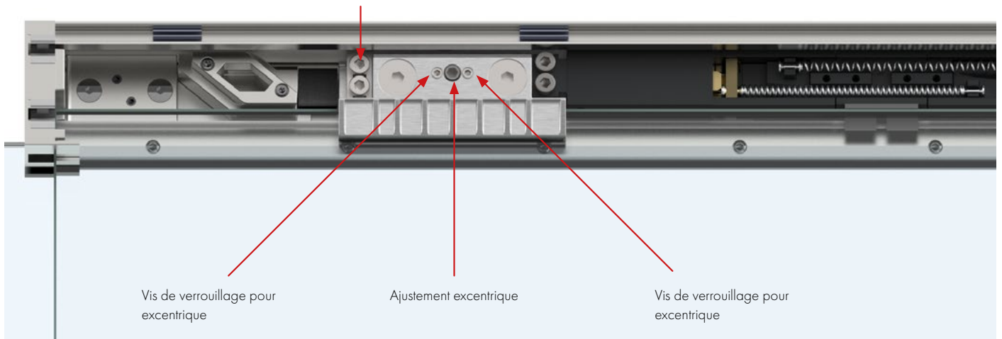
Sécurité anti lèvement
