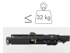
2x Softstop 1 coté (32 kg) Réf. Art.: 8822RAL7016-SSD-32
