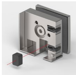
Support pour fixation sur verre latéral coté passage Réf. Art.: 8822ZN_-GL/GR
