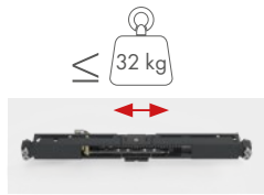
Softstop 2 cotés (32 kg) Réf. Art.: 8822RAL7016-SSDD
