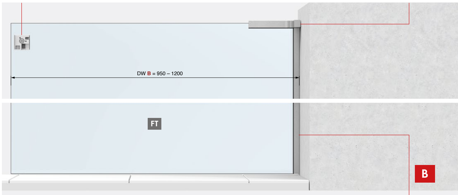
Exemple Équerre de stabilisation réglable Réf. Art.: 8439ZN_L-180
