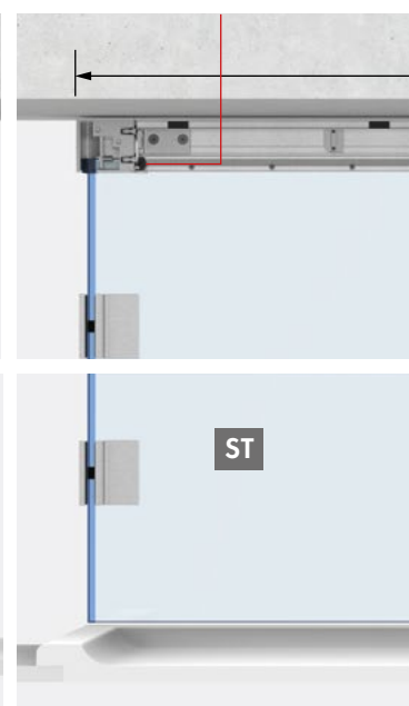
Butée dans le support mural Réf. Art.: 8822VA-AP
