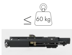
2x Softstop 1 coté (60 kg) Réf. Art.: 8822RAL7016-SSD-60
