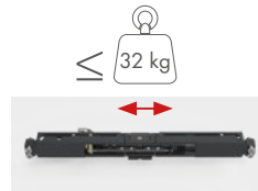
Softstop des 2 cotés (32 kg) Réf. Art.: 8822RAL7016-SSDD
