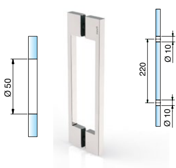
Réf. Art.: 8277MS_
