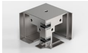
Raccord d'angle Fixe/Panneau coulissant Réf. Art.: 8822ZN_EST90
