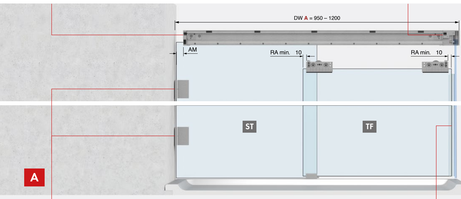
Capot latéral pour rail pincé Réf. Art.: 8822ZN_-ELST/ERST
