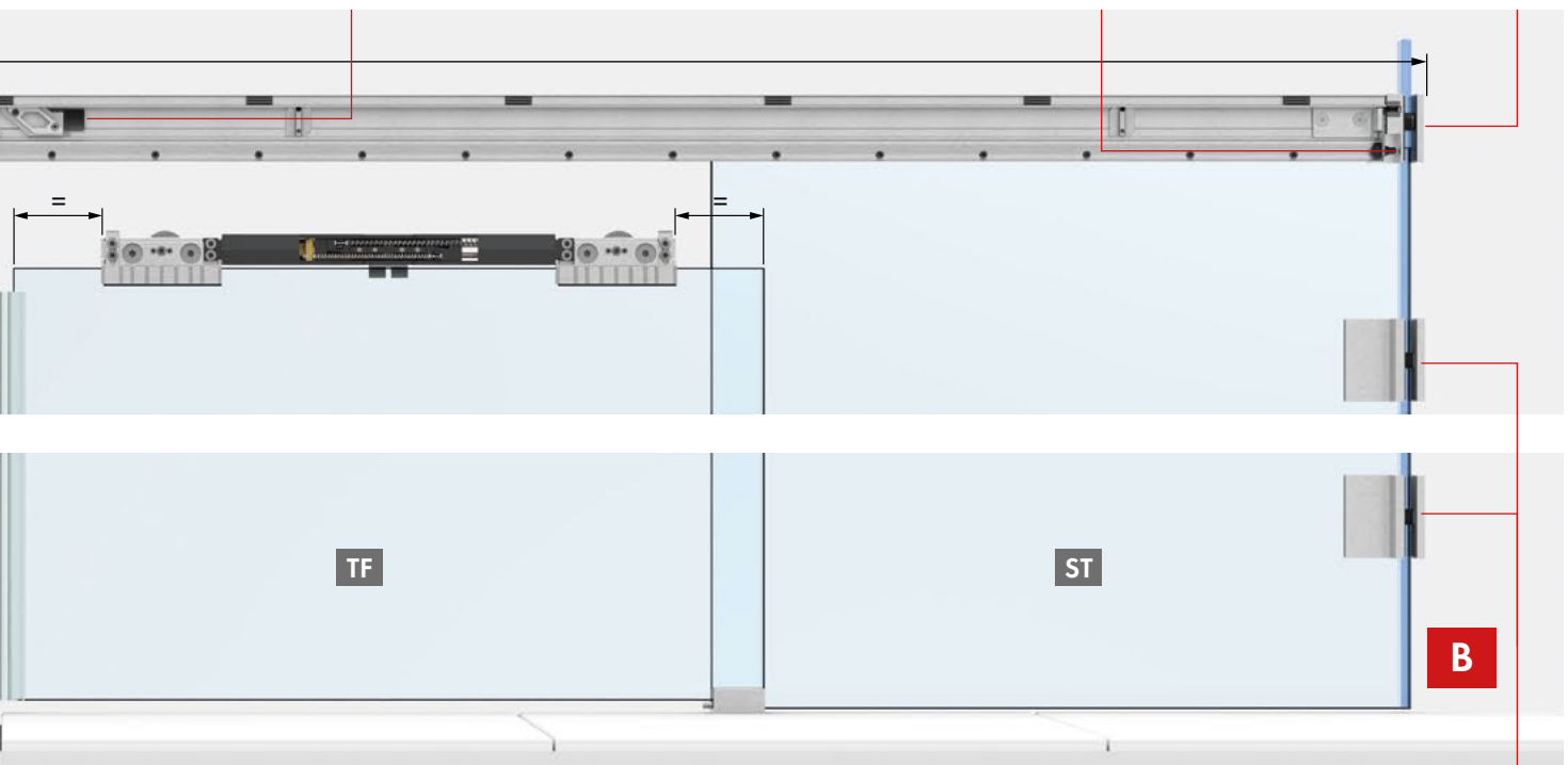
Butée dans le rail de guidage Réf. Art.: 8822ZN_-EA
