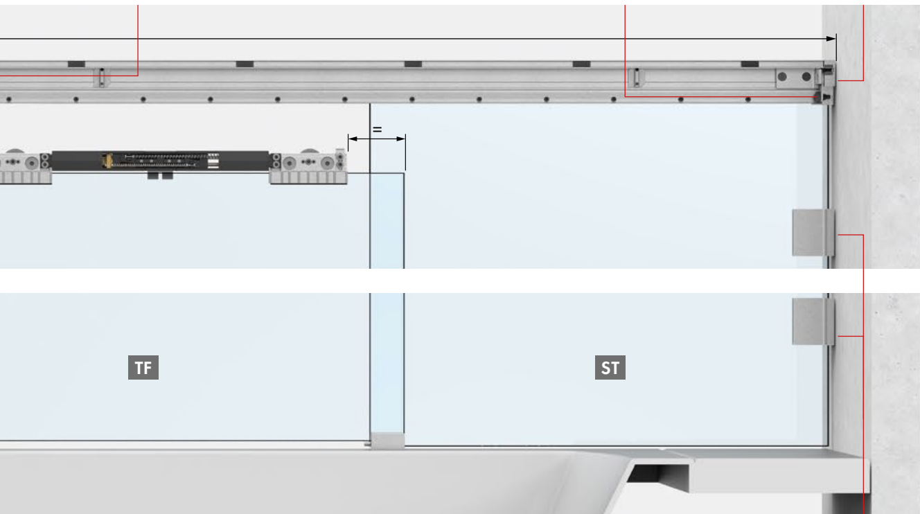
Butée dans le rail de guidage Réf. Art.: 8822ZN_EA
