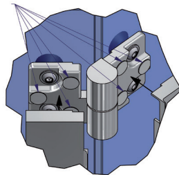
502332, doppelseitiger Klebepunkt 502332, double-sided adhesive tape
