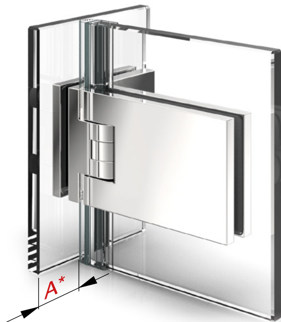
*Einrückmaß (A) am Seitenteil kann selbst bestimmt werden *offset dimension (A) on the side panel can be determined by the installer
