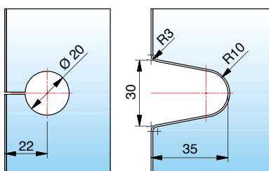
Glasbearbeitung für 6/8/10 mm, Bohrung Ø20 mm oder Randausschnitt R35 glass processing for 6/8/10 mm, hole Ø20 mm or recess R35
