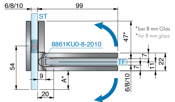
mit Dichtprofil 8861KU0-8-2010, für 8 mm Glas, Beispiel: 30 mm eingerückt with seal profile 8861KU0-8-2010, for 8 mm glass, example 30 mm set inwards
